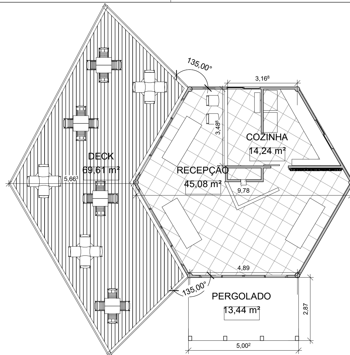
1 PAV. TÉRREO 1 : 100
